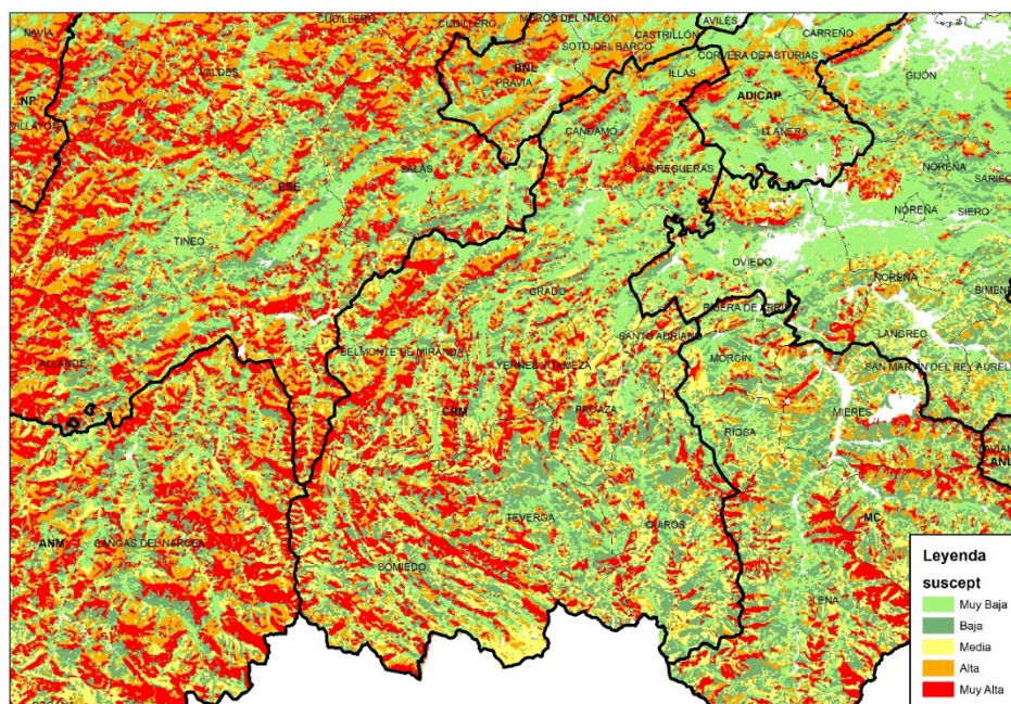
Gráfico 7. Susceptibilidad a incendios
